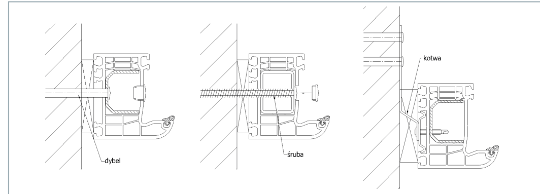
Rys. 5 Rodzaje łączników mechanicznych.
