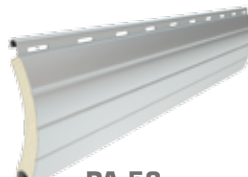
PA 52 wysokość profilu: 52 mm grubość: 13 mm
