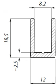
3. Profil nakładany
