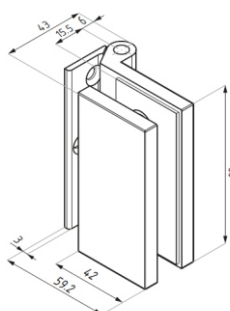
1. Zawias Simpli
