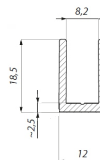
5. Profil nakładany
