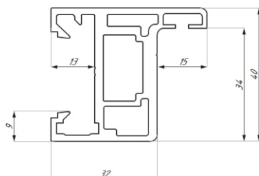
6. Zamek Rolkowy
